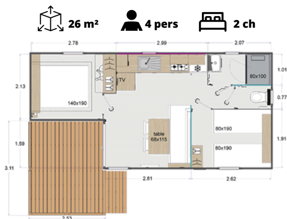
COTTAGE 2 CHAMBRES
